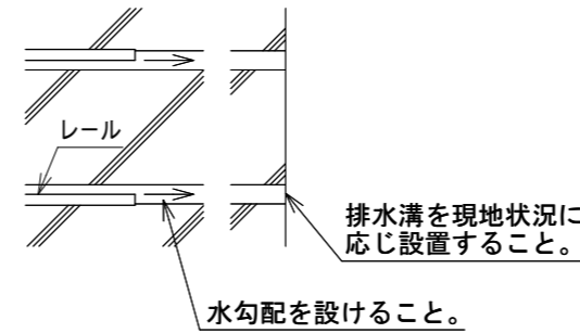
レール端部コンクリート処理図
