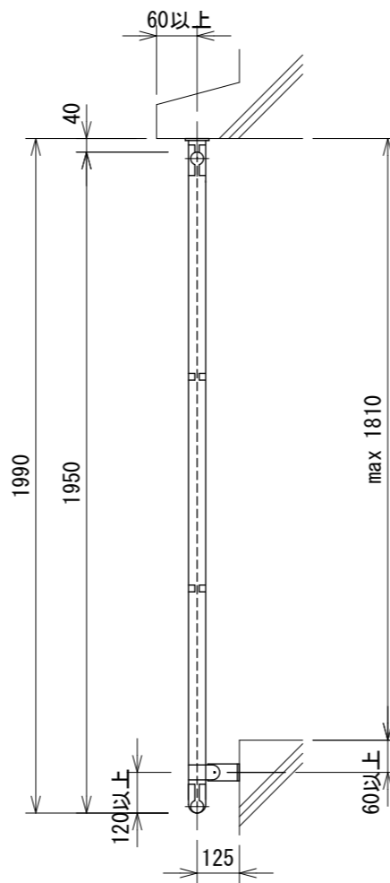
胴縁に金網取付断面図 S=1:3
