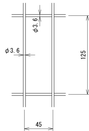
Wメッシュ S=1:3 芯径を示す
