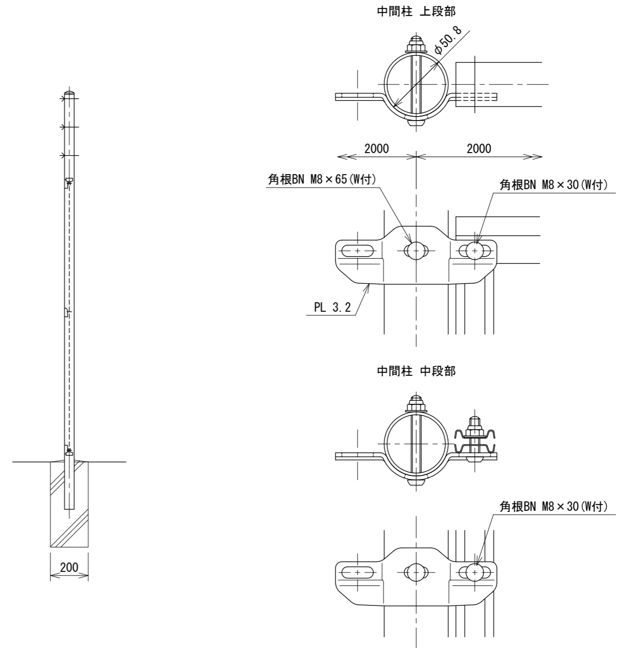
パネル取付図 S=1:3
